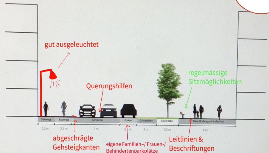
Straßenquerschnitt A (1:200)
